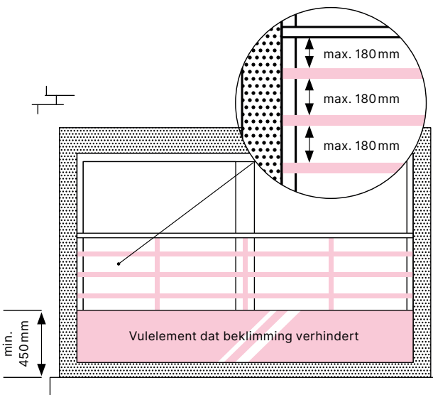
fig. 2 Openingen tussen de horizontale borstweringselementen in mm.
